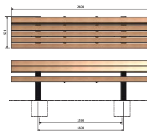
96.102.200 TopfBalk 30x30x30 mit 2 M10x60 h.u.h. 160 mm 2x
