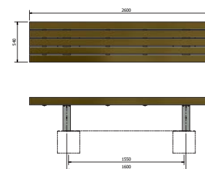
96.102.200 TopfBalk 30x30x30 mit 2 M10x60 h.u.h. 160 mm 2x
