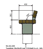
96.102.200 TopfBalk 30x30x30 mit 2 M10x60 h.u.h. 160 mm 2x
