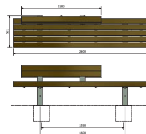
96.102.200 TopfBalk 30x30x30 mit 2 M10x60 h.u.h. 160 mm 2x
